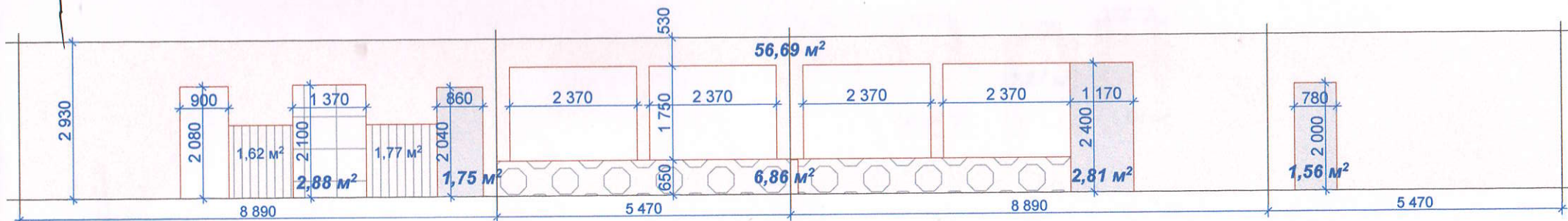
Розгортка стін
